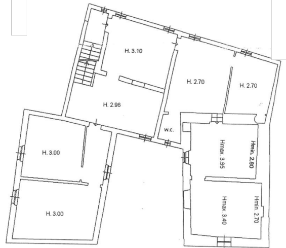
PIANO PRIMO
