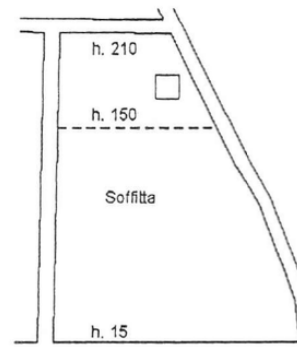
Pianta Piano Sottotetto
