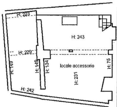
SECONDO PIANO SOTTOSTRADA
