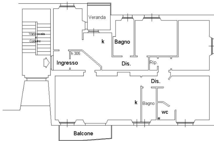
PIANO PRIMO
