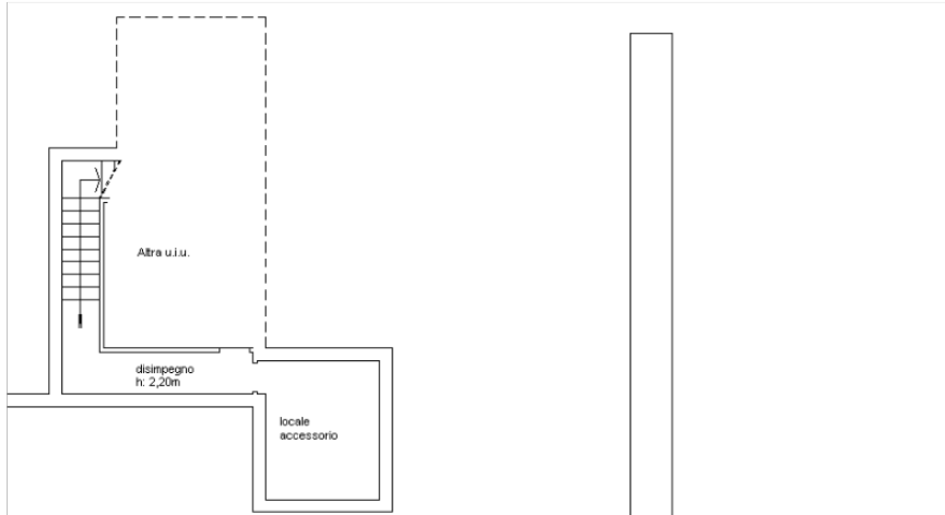
PIANO PRIMO SOTTOSTRADA
