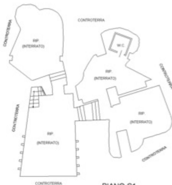
PIANO S1 ALTEZZA INTERNA H 3.95 m
